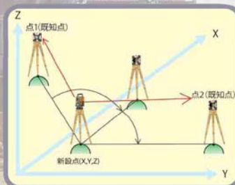
【2点後方交会法】
