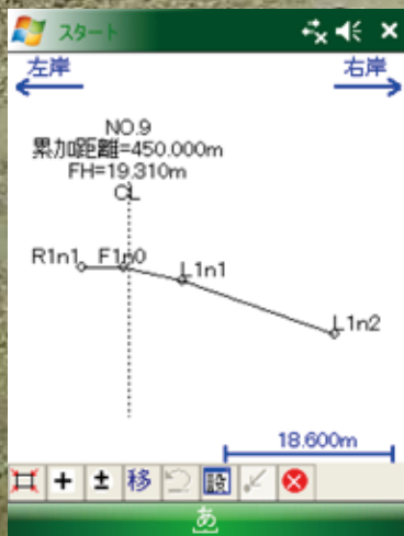
横断平面図
