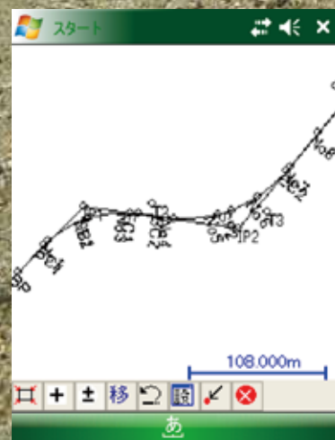
平面線形
